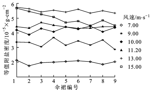
(a)ESDD 测量结果
