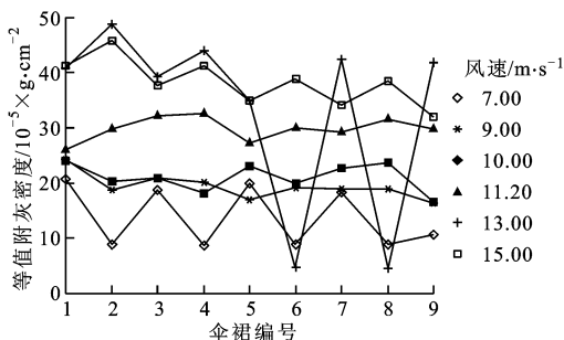
(b)NSDD 测量结果
