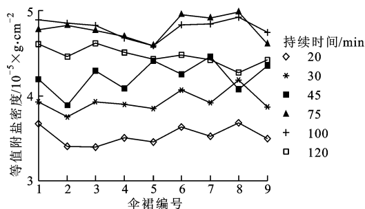
(a)ESDD 测量结果
