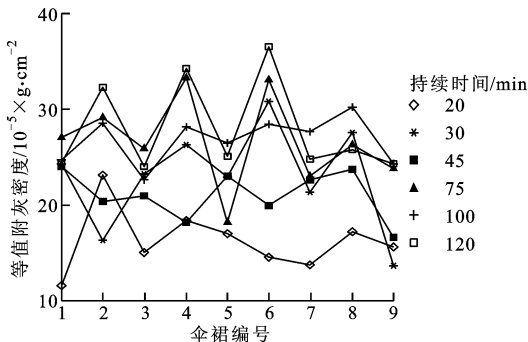
(b)NSDD 测量结果
