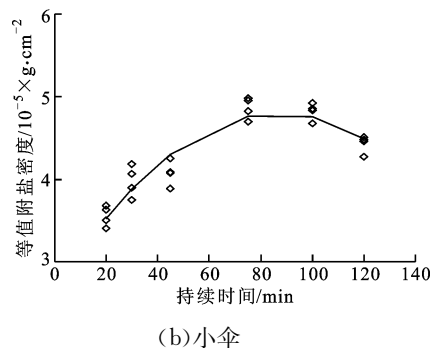
图6 伞裙上表面平均盐密和时间的关系
